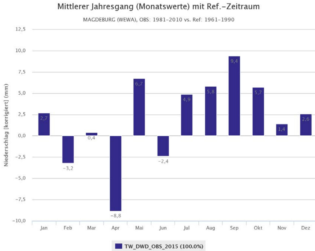
Abbildung 15: gemessene Niederschlagsänderung an der DWD-Station Magdeburg, Quelle:rekis.org
