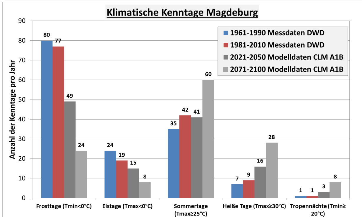
Abbildung 14: Klimatische Kenntage für Magdeburg (eigene Darstellung, Daten:rekis.org)
