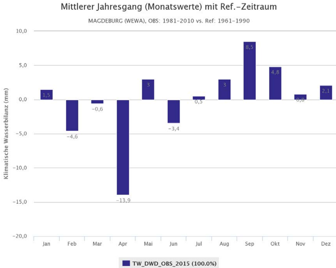
Abbildung 19: gemessene Änderung der Klimatische Wasserbilanz an der DWD-Station Magdeburg, Quelle:rekis.org
