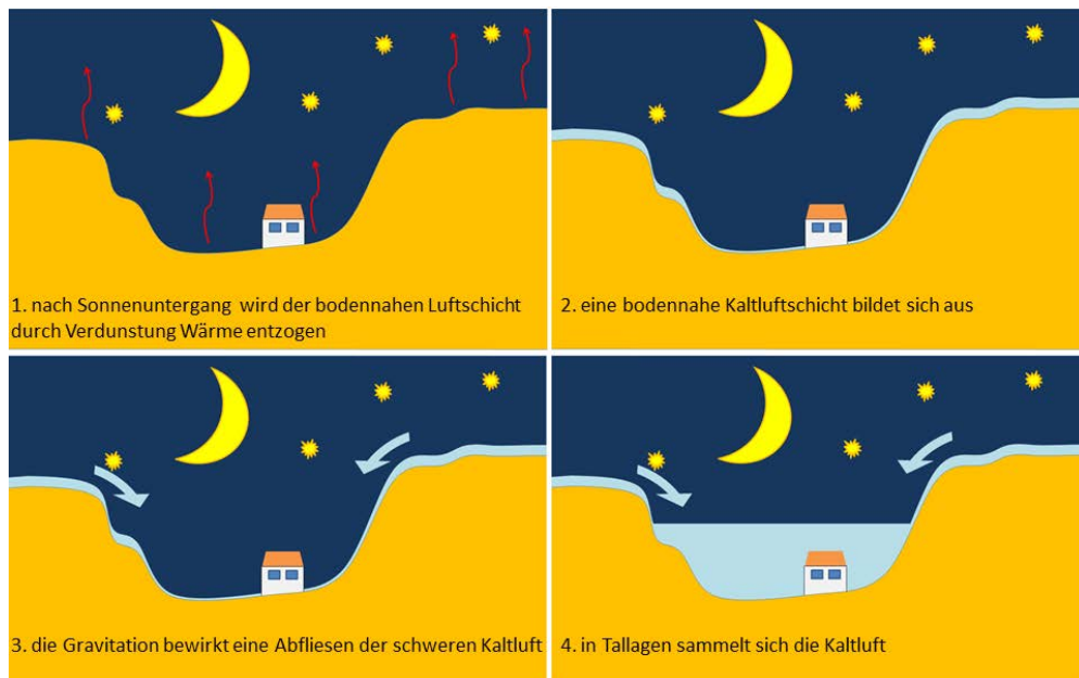
Abbildung 8: Schematische Darstellung der Kaltluftströmung (eigene Darstellung)
