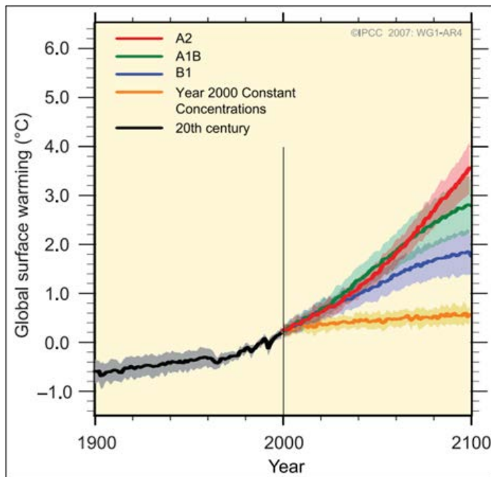
Abbildung 2: Veränderung der mittleren globalen Lufttemperatur für verschiedene Emissionsszenarien (Quelle: IPCC 2007a, verändert)
