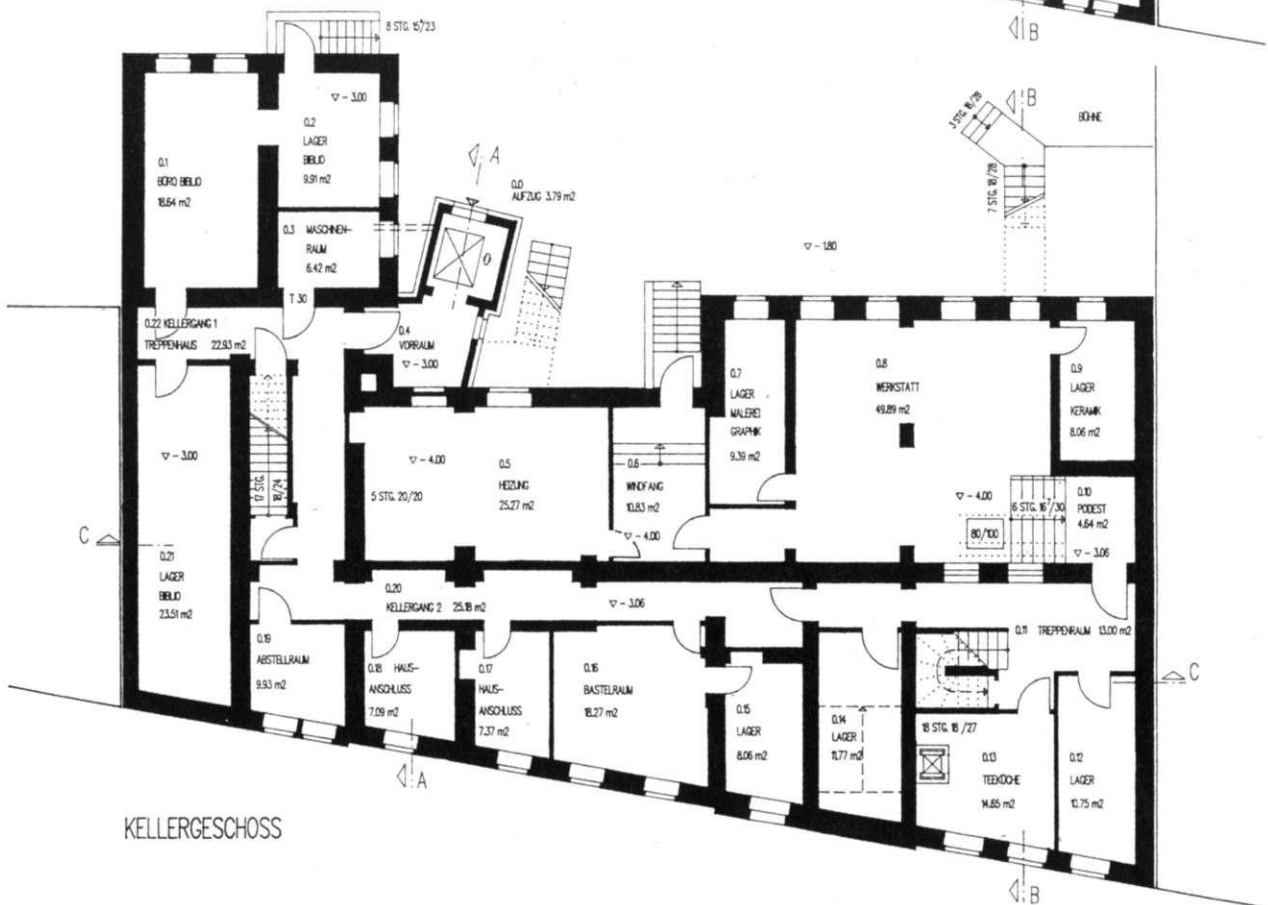
ERDGESCHOSS
