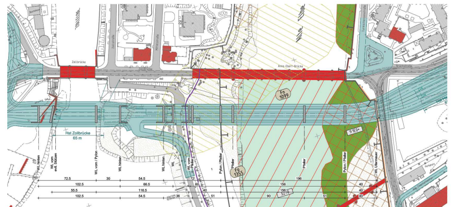
GRUNDRISS (VARIANTEN ZUSAMMENGEFASST)
